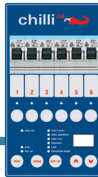
Chilli Junior Bedienfeld mit Sicherungsautomaten Panel with circuit breakers
